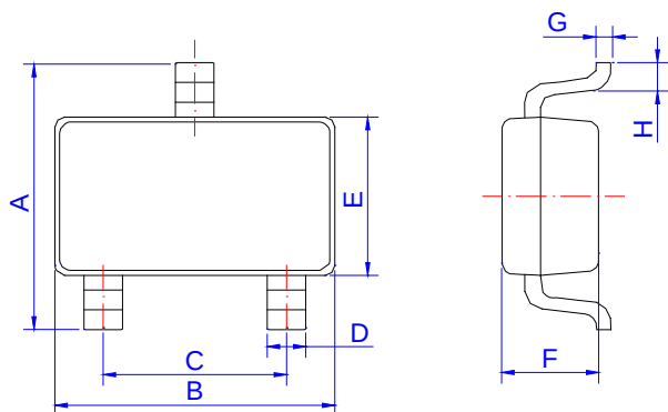
SOT-23-3L
